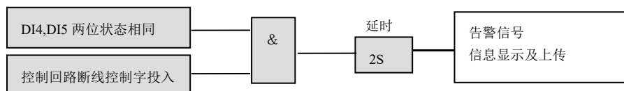
图 3-13 控制回路断线原理框图
