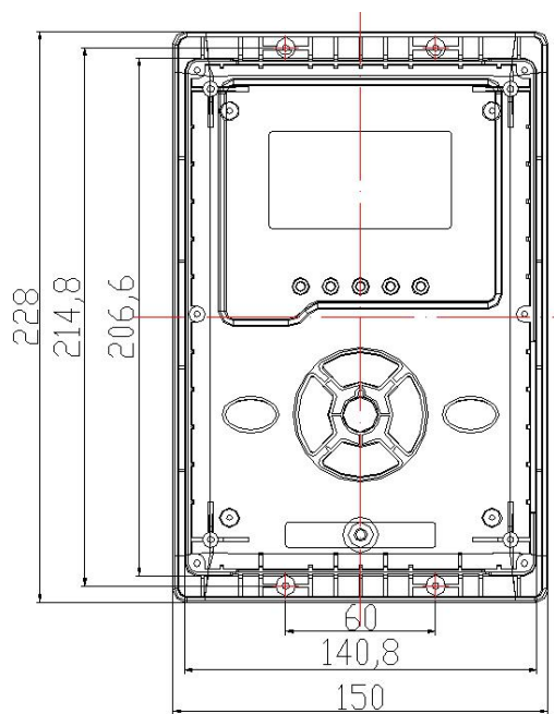
图 5-1 装置正视图
