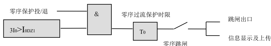
图 3-5 定时限零序过流保护原理框图
