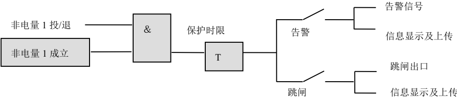
图 3-14 非电量保护原理框图
