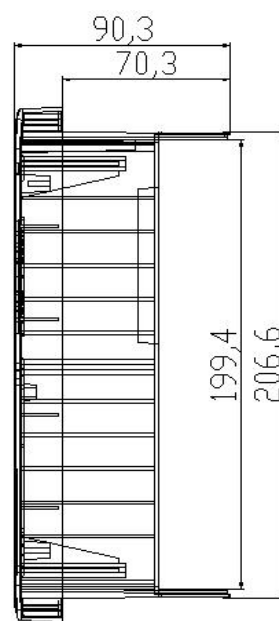
图 5-2 装置侧视图
