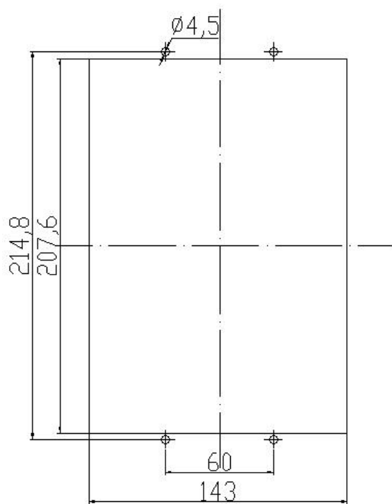
图 5-1 装置正视图
