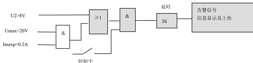
图 3-12 PT 断线监视原理框图
