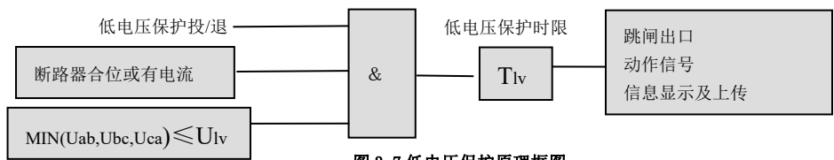
图 3-7 低电压保护原理框图
